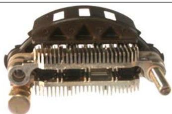
137861 Rectifier
