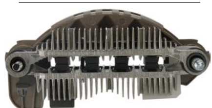
239995 Rectifier
