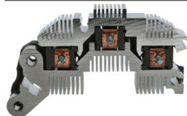
232069 Rectifier
