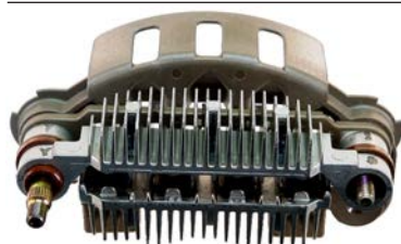
230046 Rectifier
