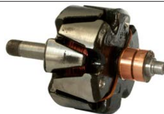
231293# Rotor
