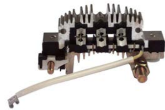
139518 Rectifier
