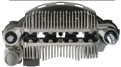
333056 Rectifier
