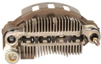
233483 Rectifier
