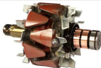
230869 Rotor
